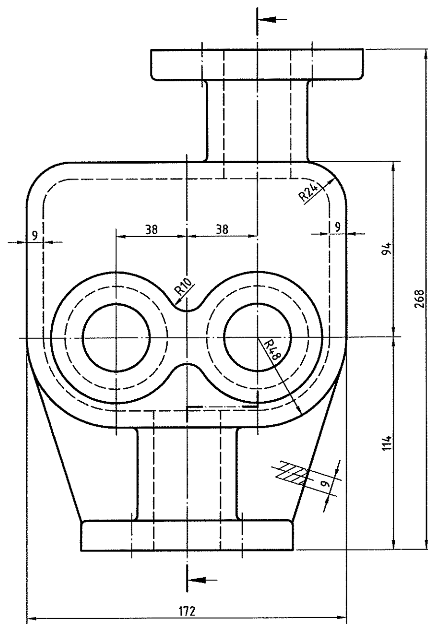
前視圖
