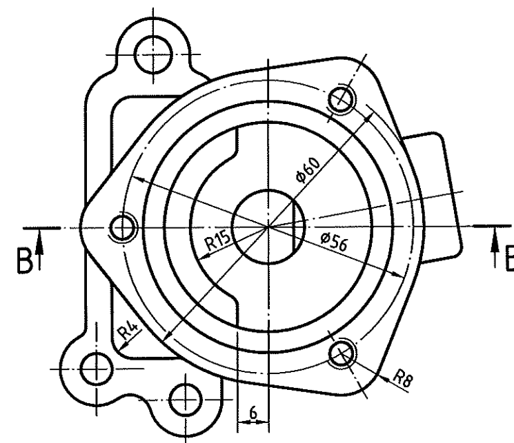
A 視圖
