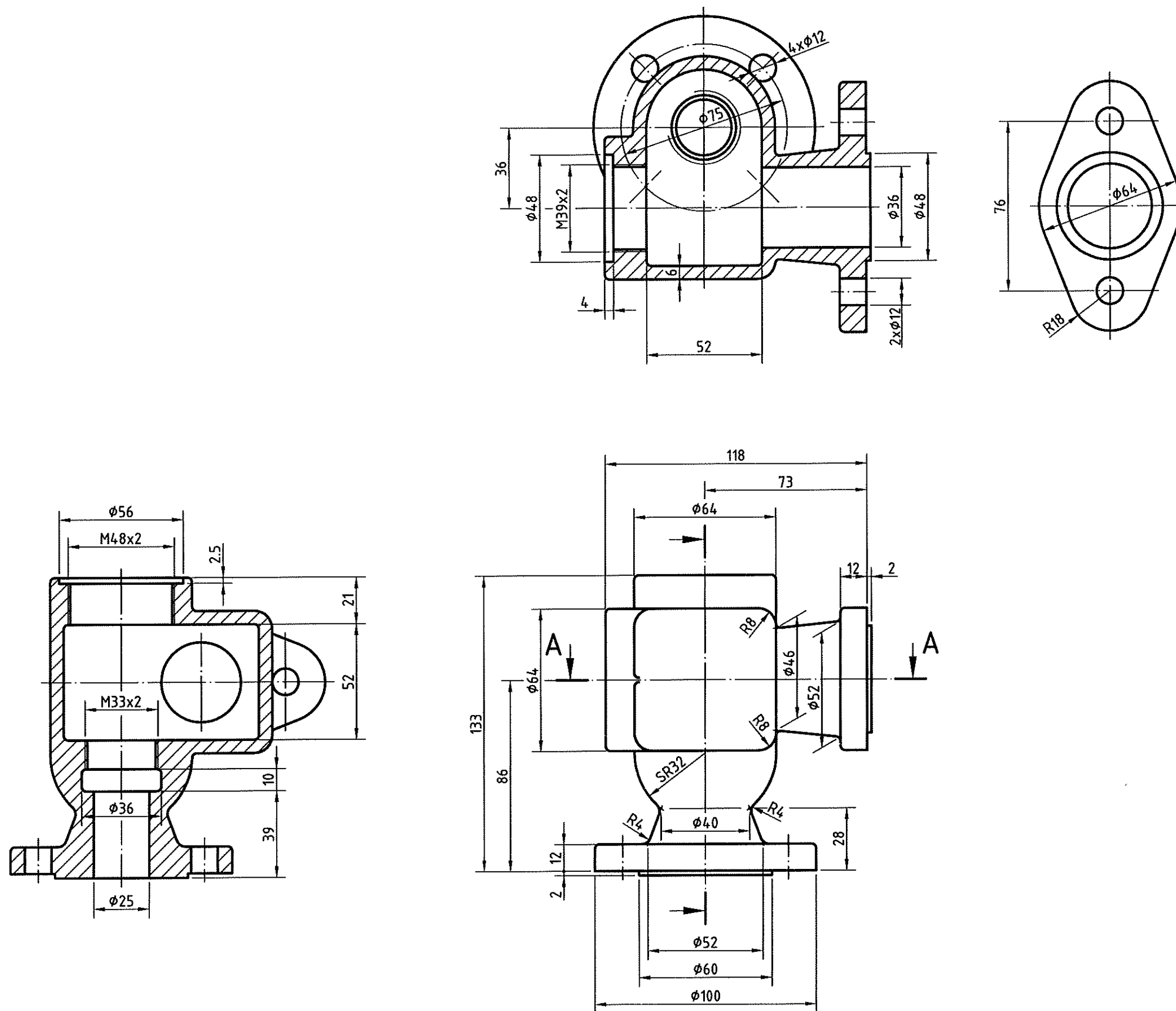
前視圖
