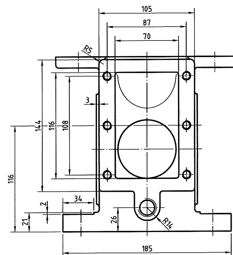
A-A剖面
