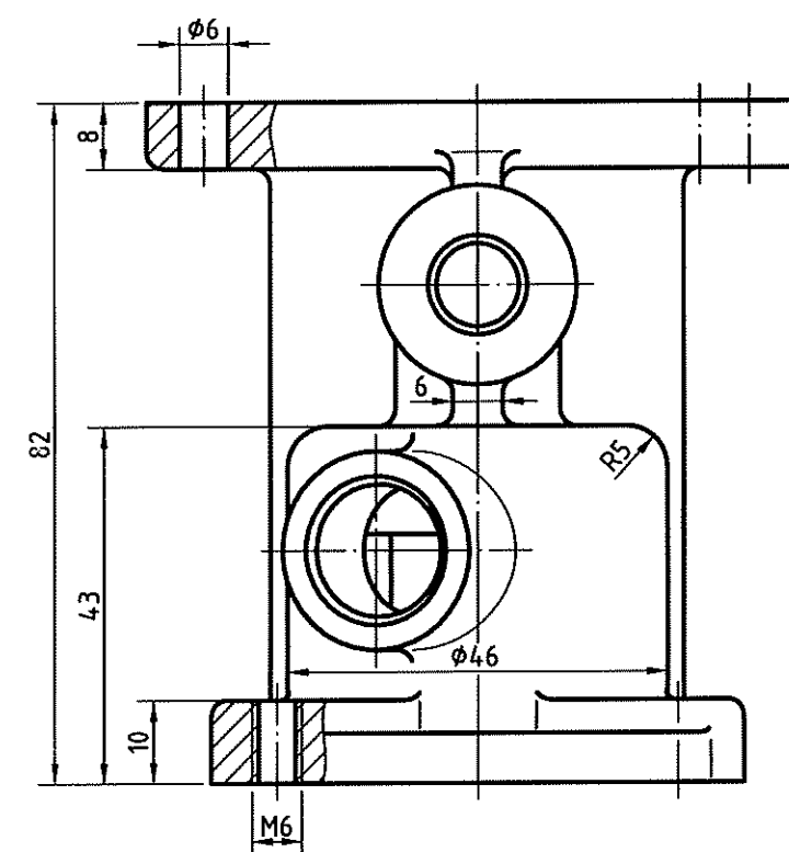
A 視圖
