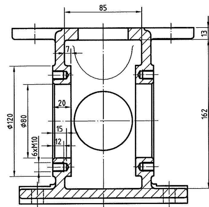
A-A剖面
