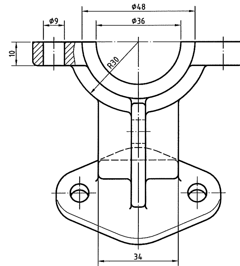
前視圖
