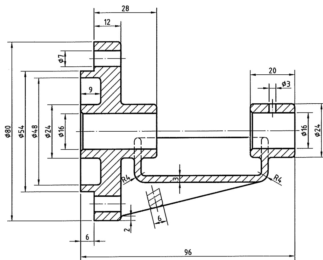
前視圖
