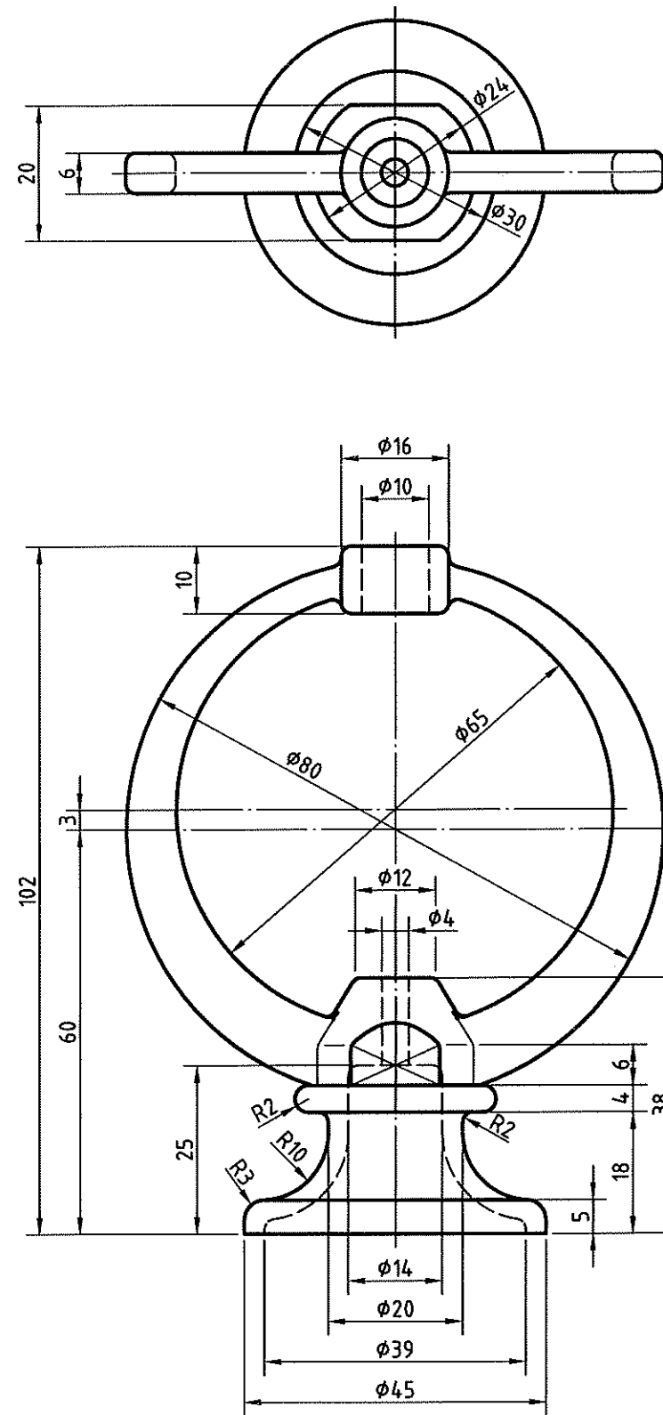
前視圖
