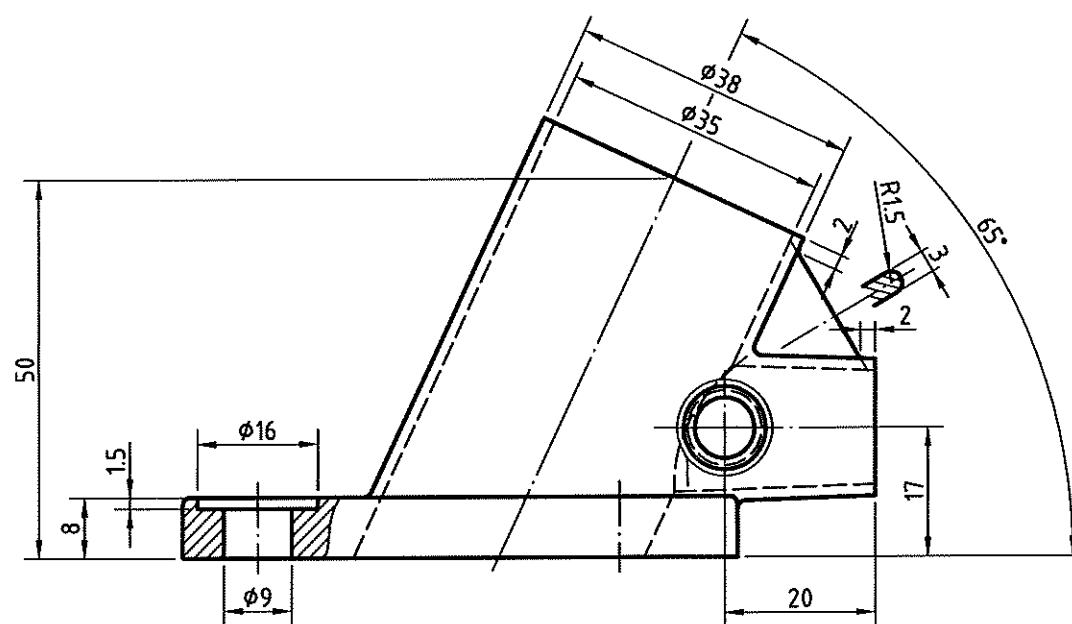
前視圖
