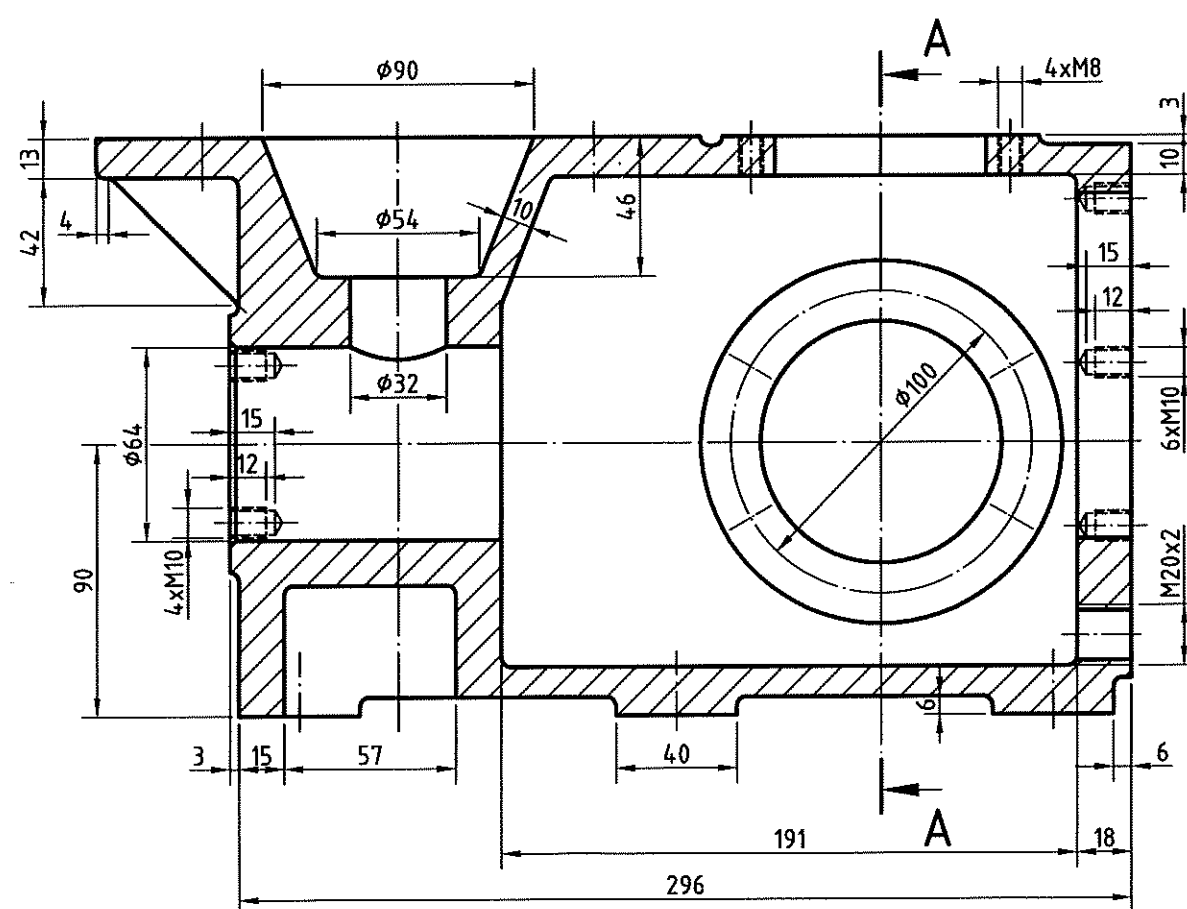
前視圖
