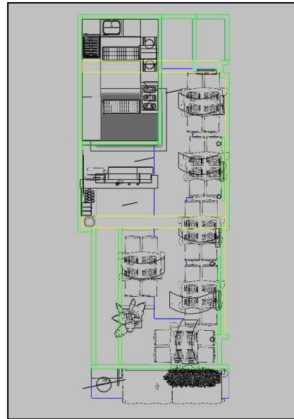
輪廓平面圖
