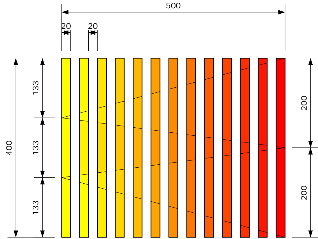
正立面圖
