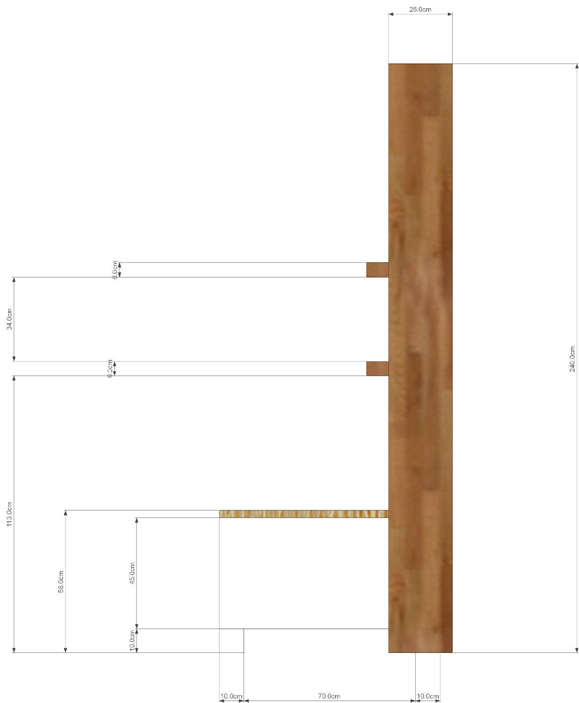
側視圖
