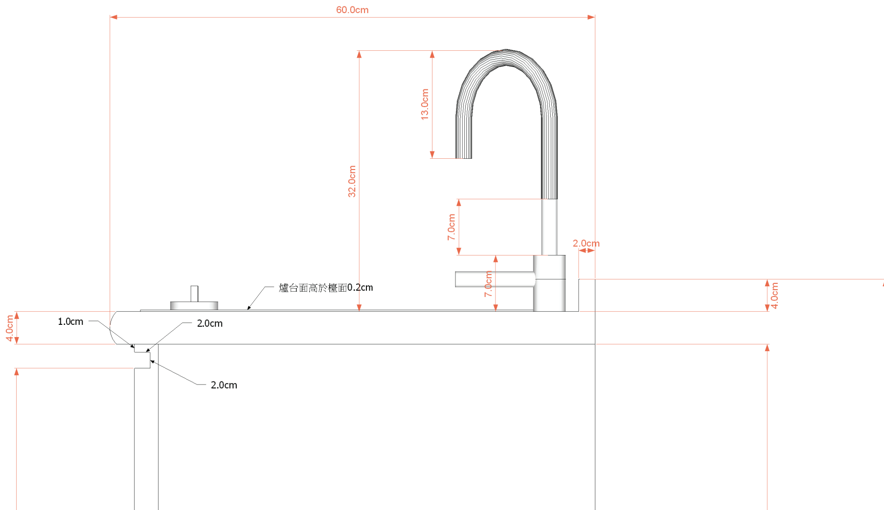
水龍頭詳圖
