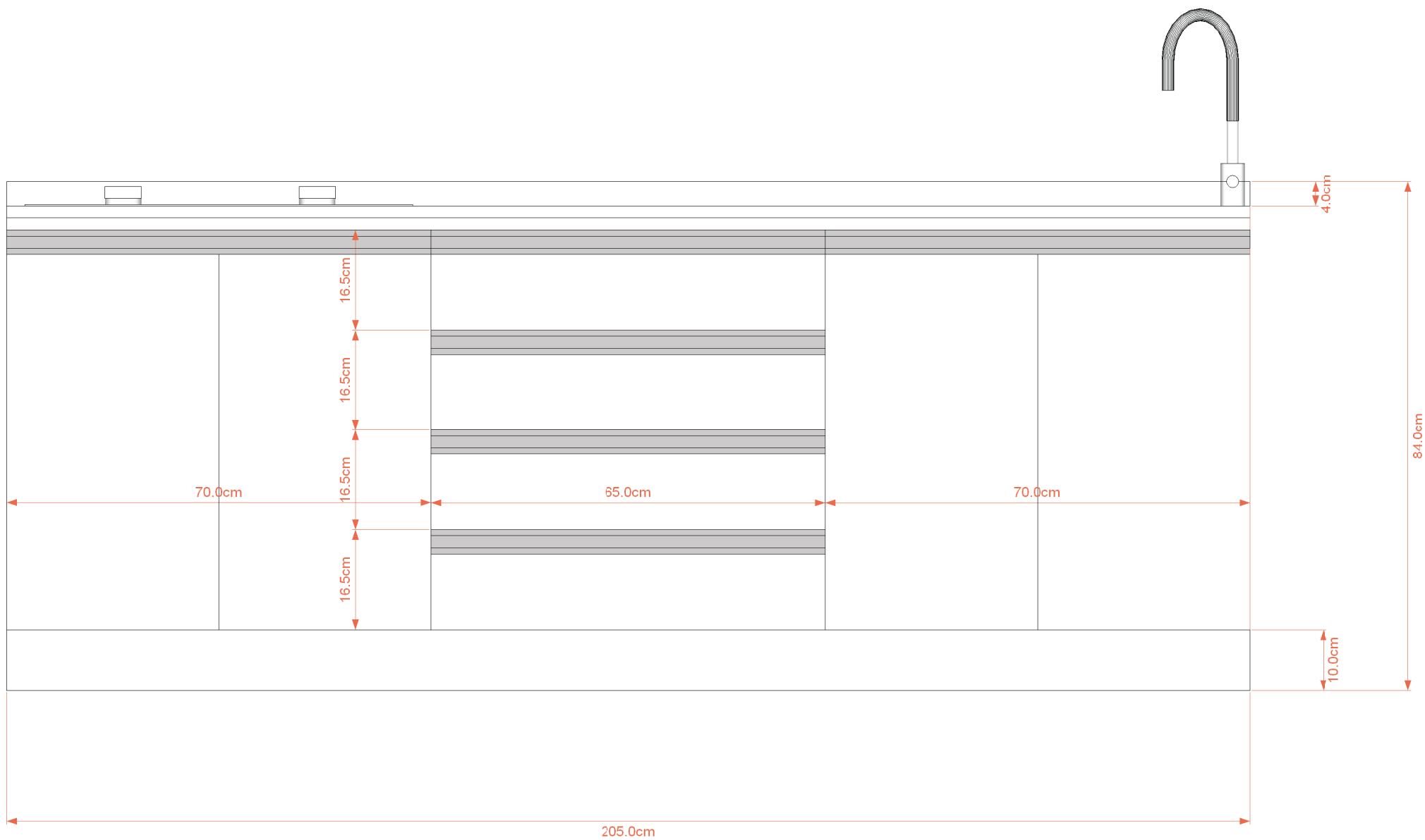
正立面圖
