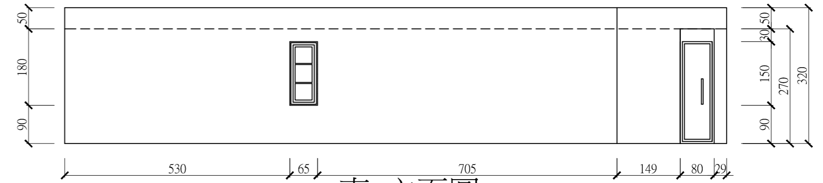
東_立面圖
