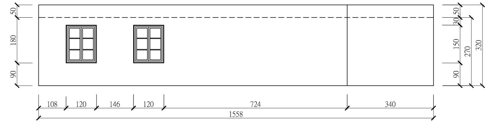
西_立面圖
