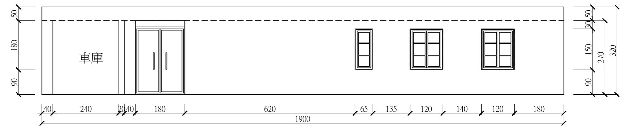
南_立面圖
