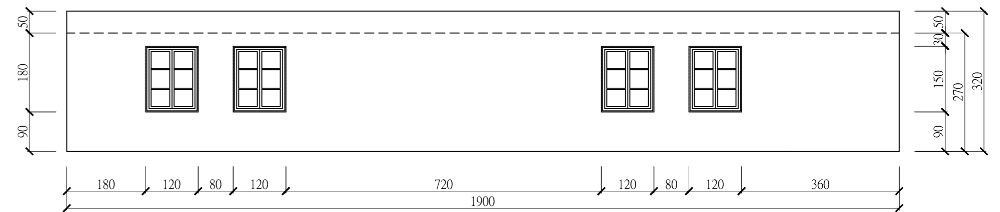
北_立面圖
