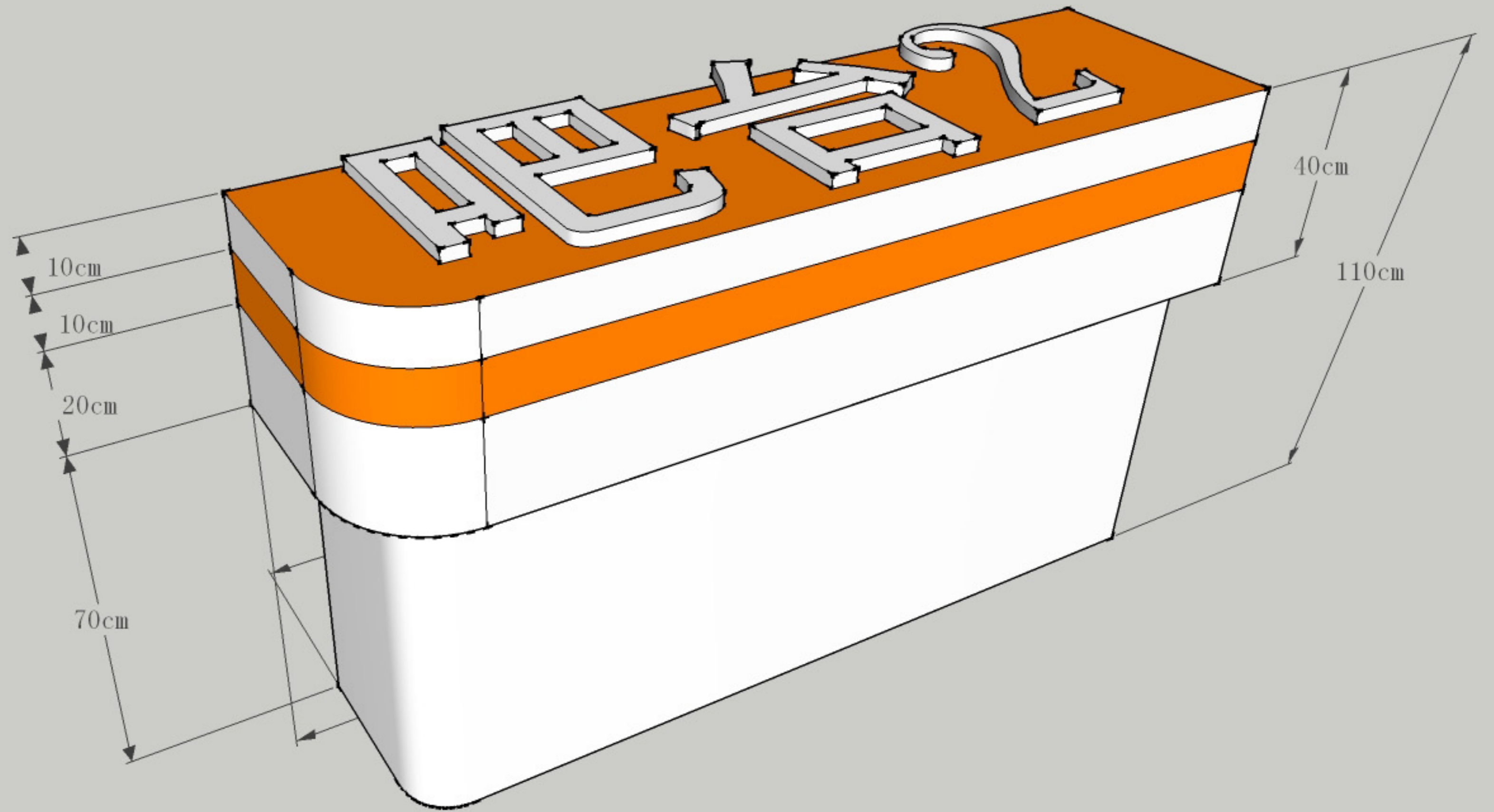
吧台2_前面尺寸圖
