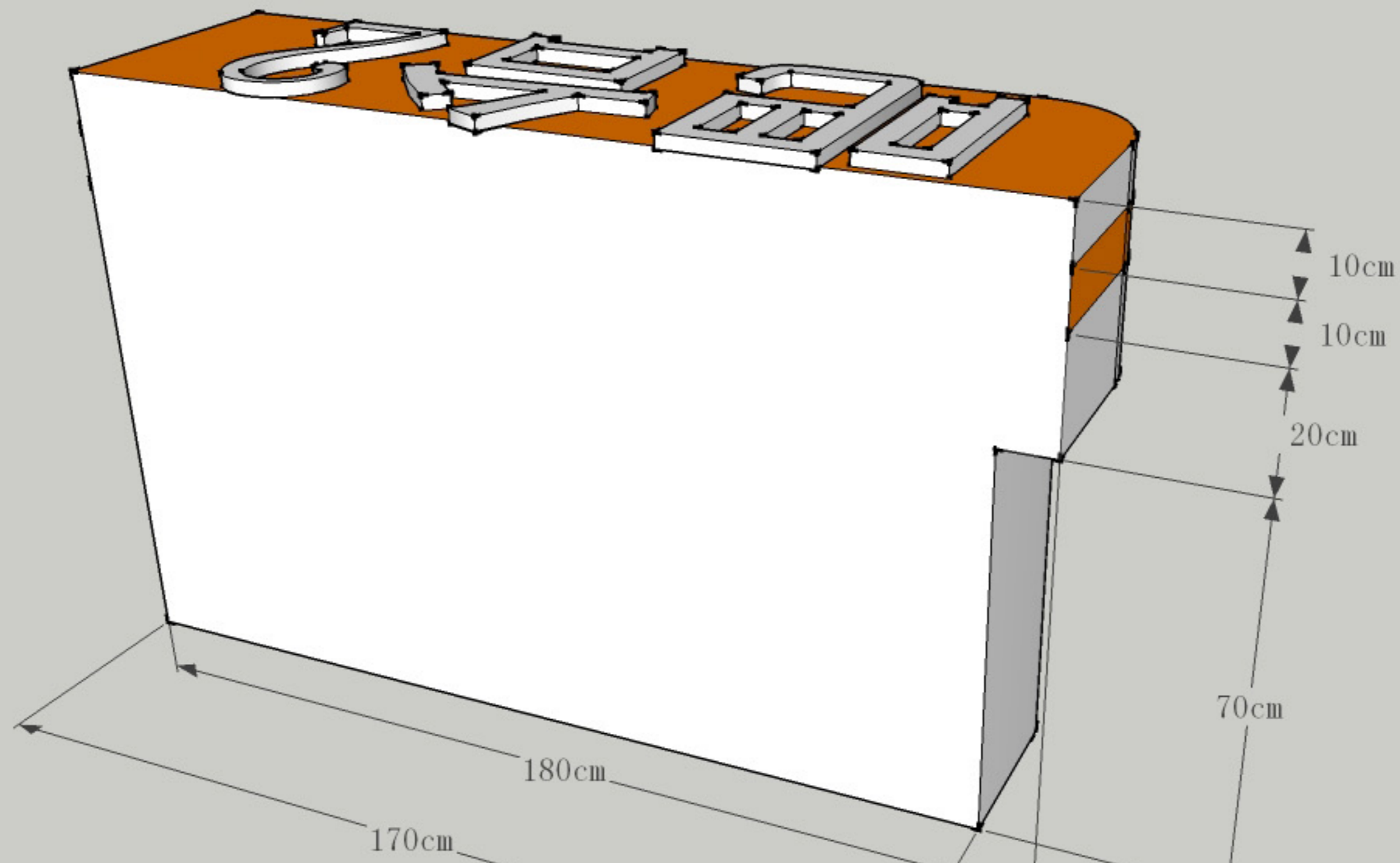
吧台2_後面尺寸圖
