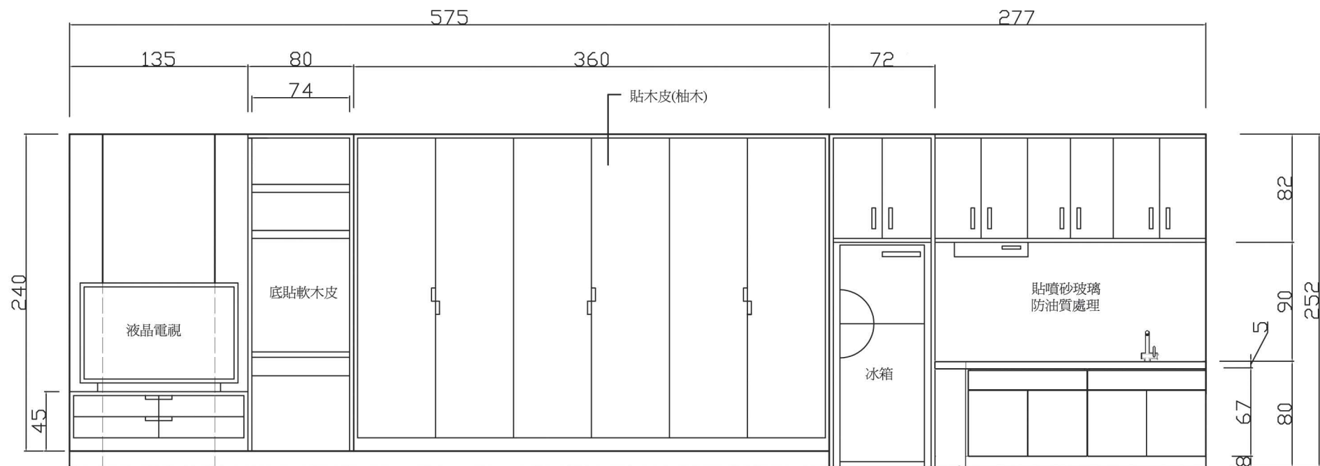
A向立面圖 SCALE 1/40
