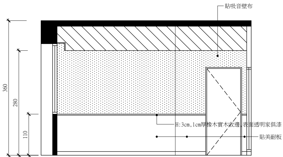
3 B204 A向立面圖 Unit=cm
