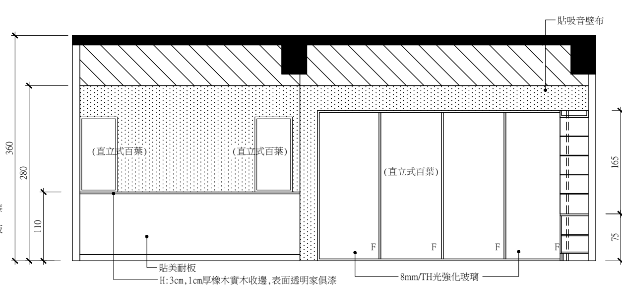
4 B204 B向立面圖 Unit=cm
