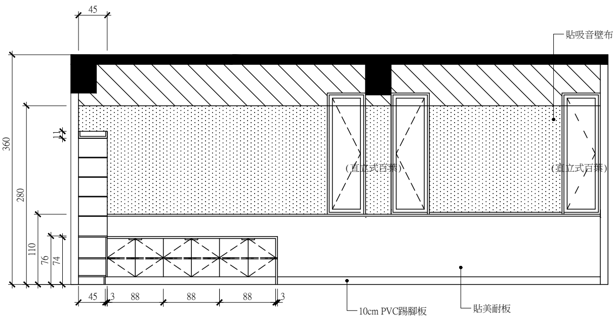
6 B204 D向立面圖 Unit=cm
