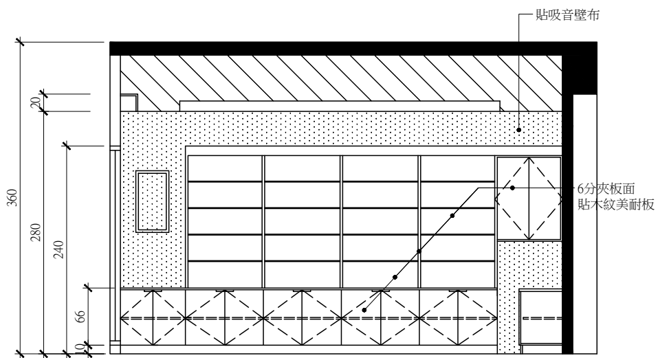
5 B204 C向立面圖 Unit=cm(主牆面)
