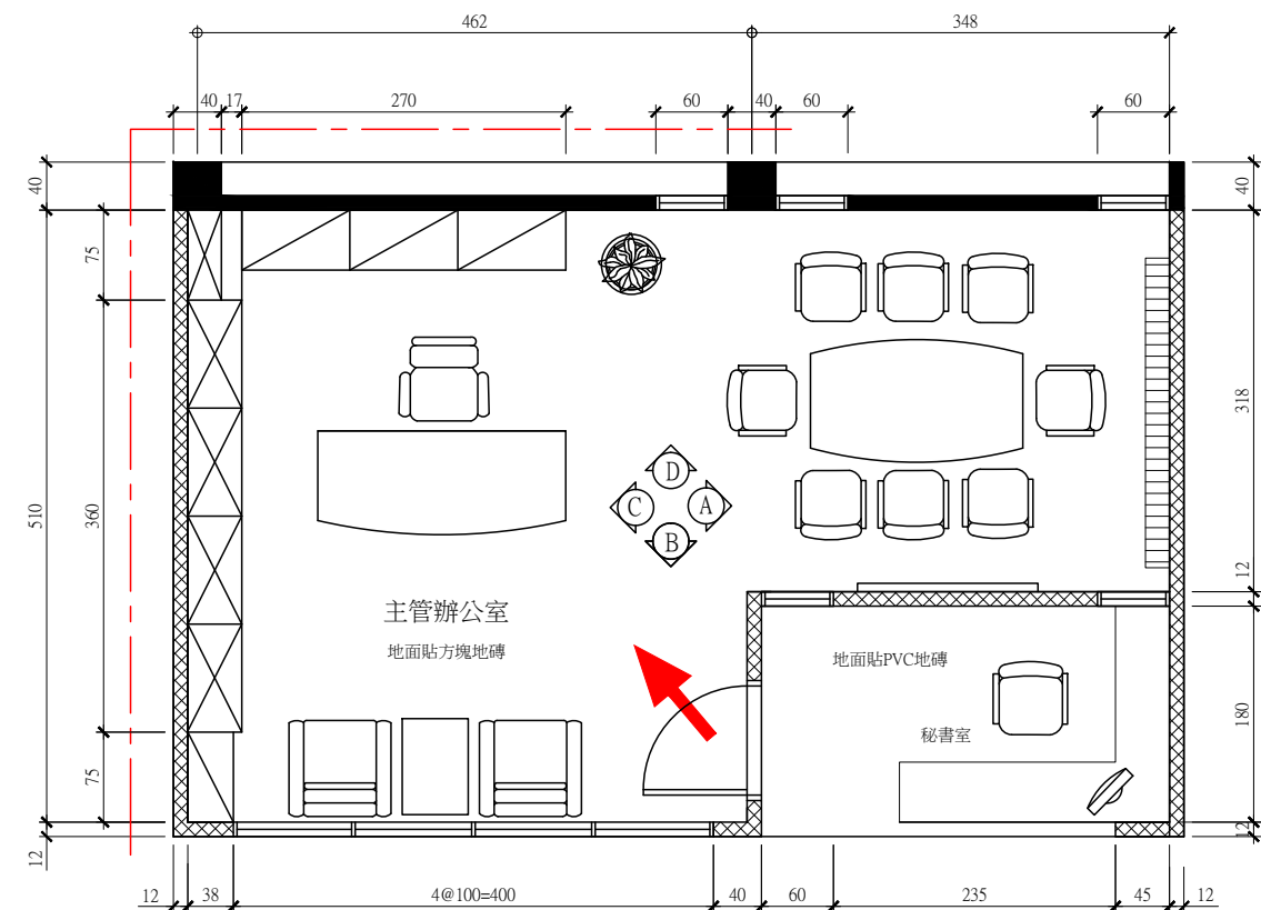
1 B204 平面圖 Unit=cm
