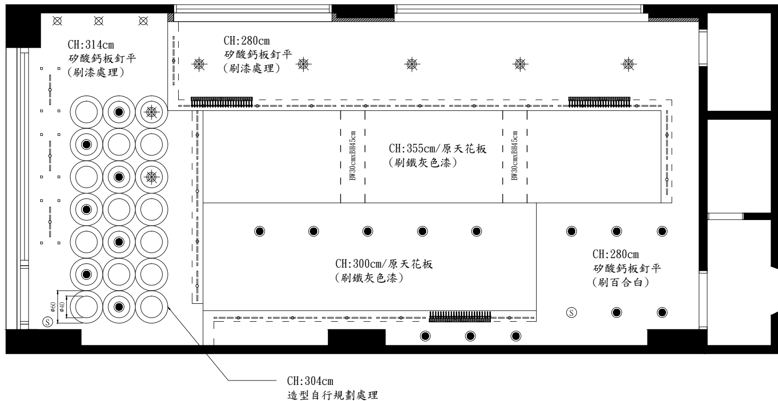
烘焙坊天花板配置圖
