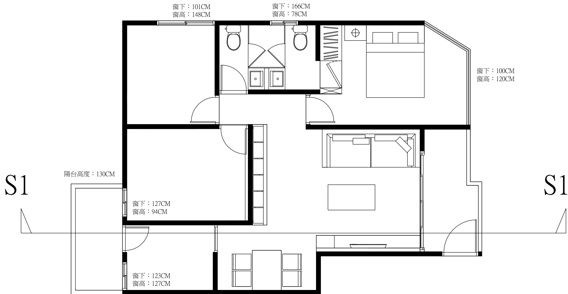
平面圖
