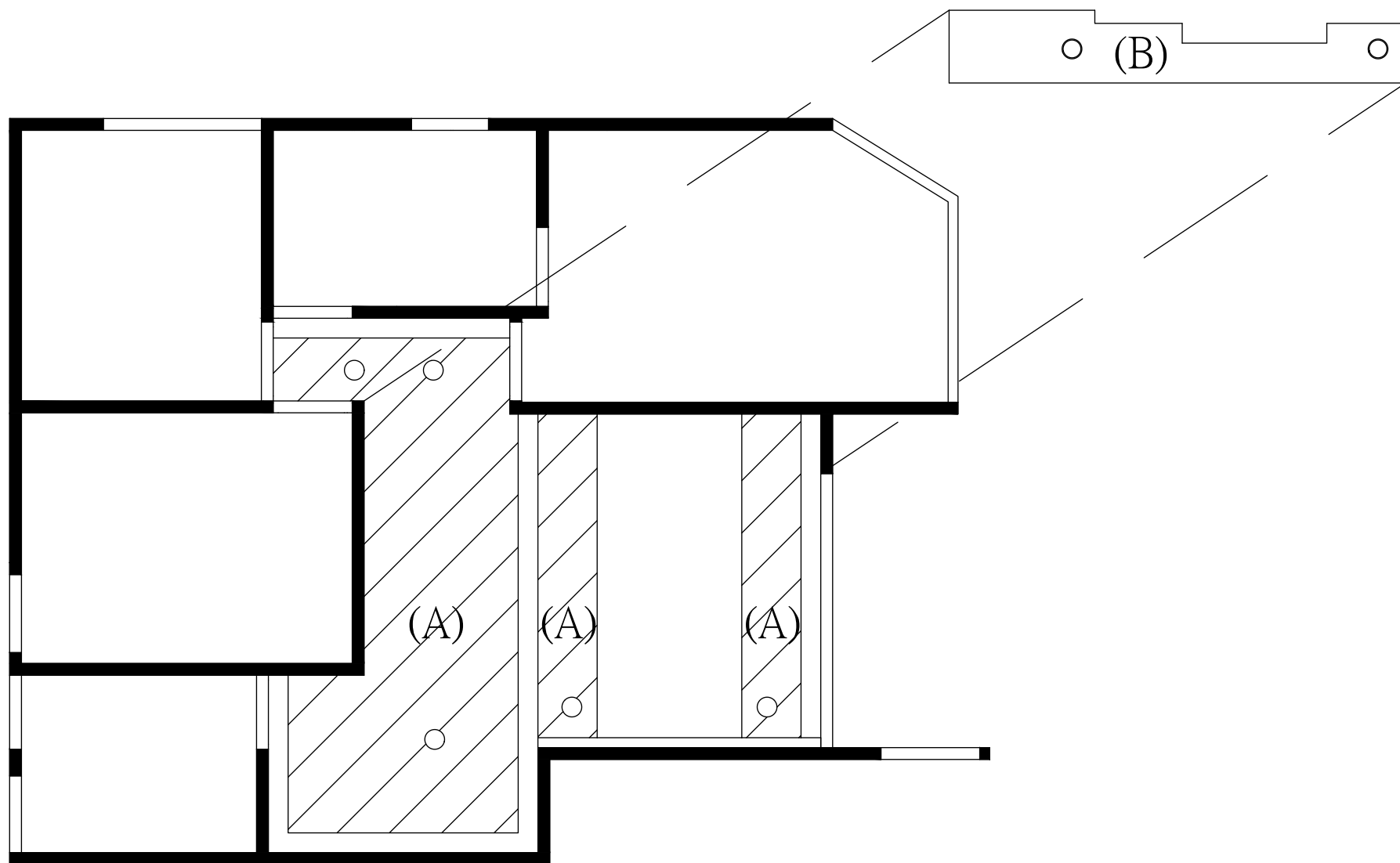
天花板平面圖
