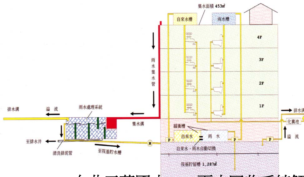
台北三芝國小 雨水回收系統解說圖
