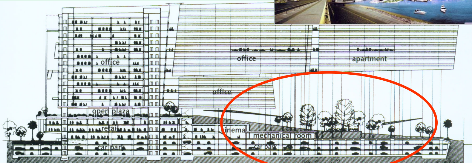
section A-A
